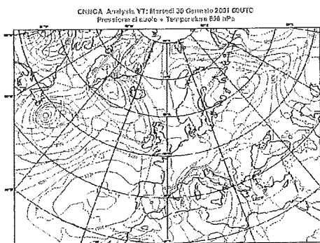
Carta dell'analisi attuale al suolo e isoterme a 850hpa
